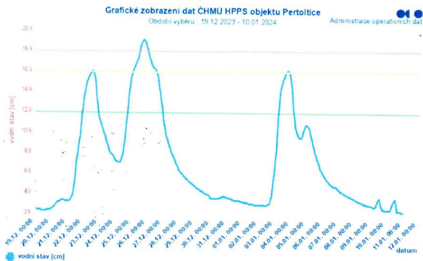
Průběh povodňové vlny na Panenském potoce ve stanici Pertoltice
